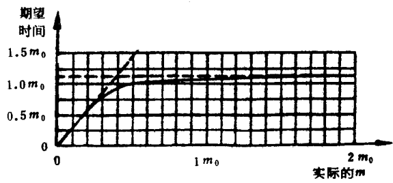
图 36 试验方案 5:4 判定的期望相关试验时间
