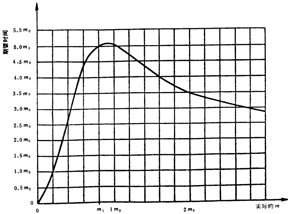
图 30 试验方案 4 : 10 工作特性曲线
