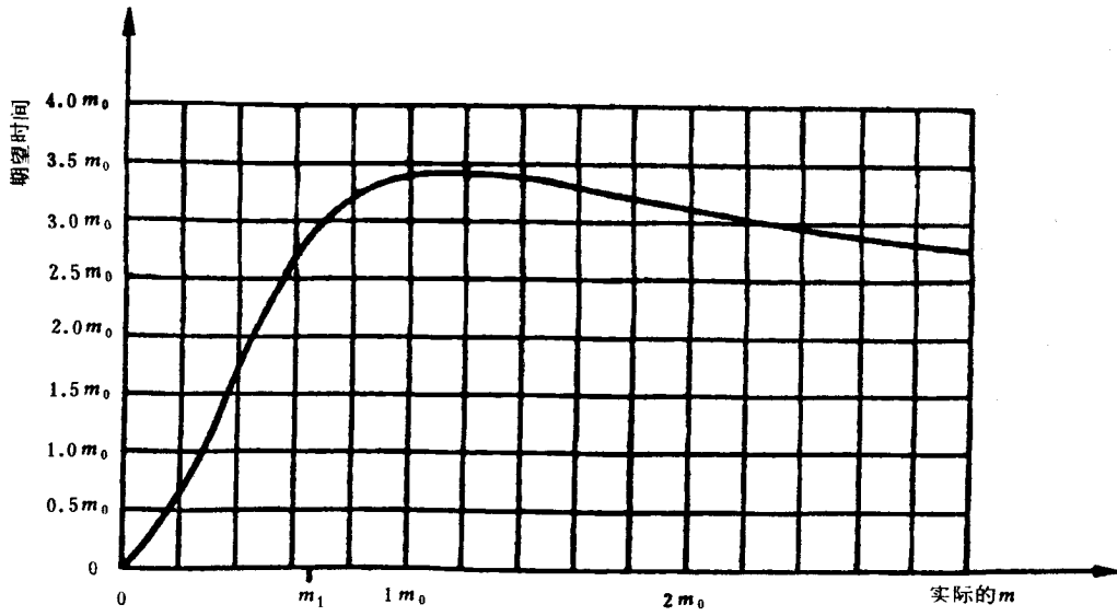
图 24 试验方案 4:8 工作特性曲线
