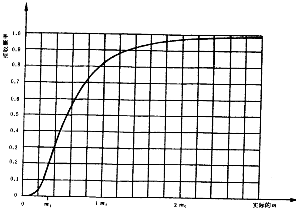
图 21 试验方案 4 : 7 工作特性曲线
