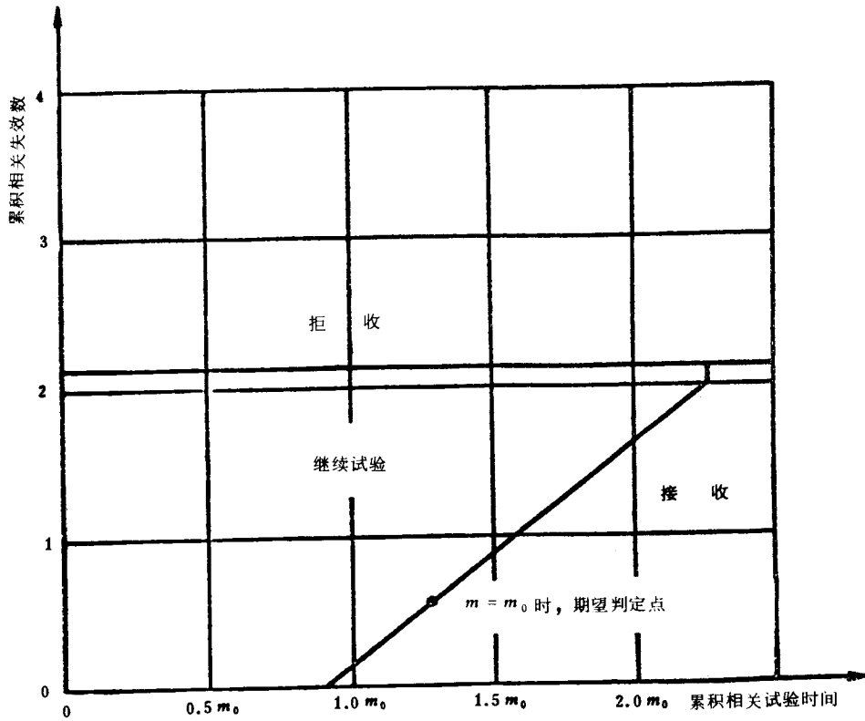
图 26 试验方案 4 : 9 ( \alpha=0.30, \beta=0.30, D_m=2.0 )
