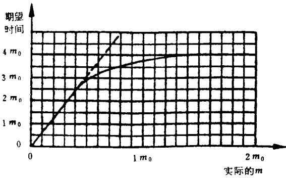
图 38 试验方案 5 : 5 判定的期望相关试验时间
