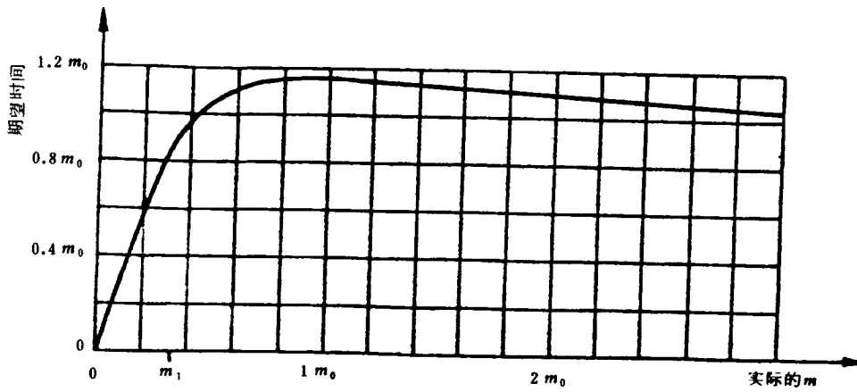
图 21 试验方案 4 : 7 工作特性曲线
