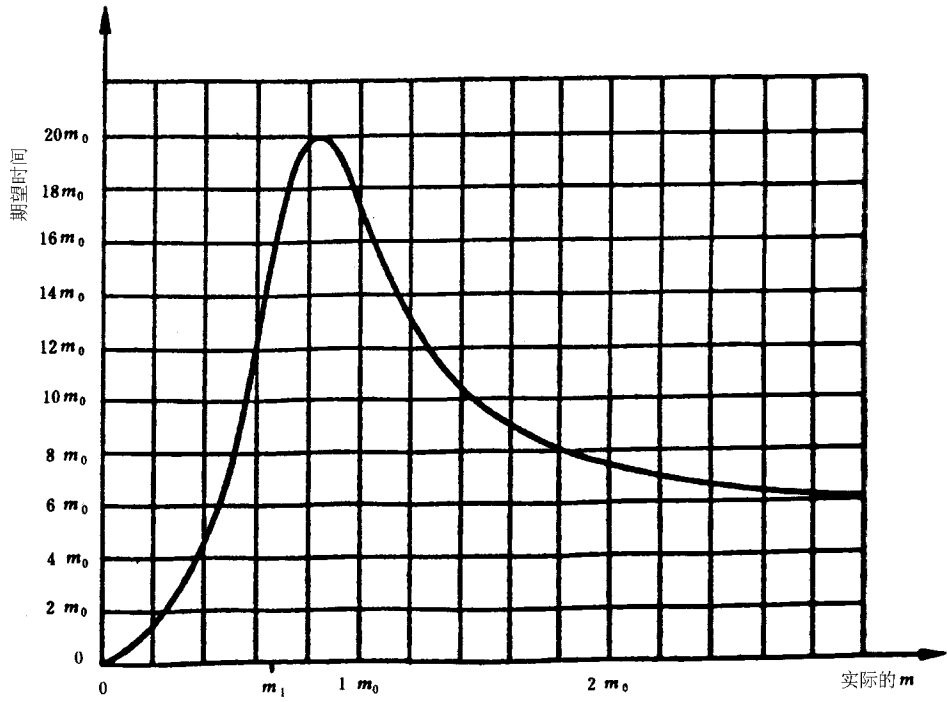
图 4 试验方案 4 : 1 判定的期望相关试验时间
