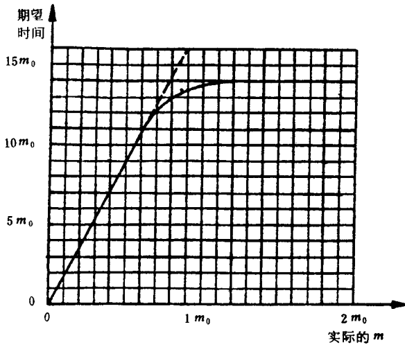
图 37 试验方案 5 : 5, 5 : 6, 5 : 7 工作特性曲线
