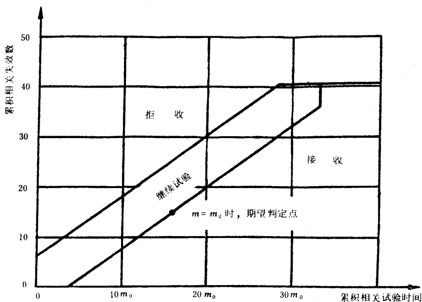
图 2 试验方案 4 : 1 ( \alpha=0.10, \beta=0.10, D_m=1.5 )
