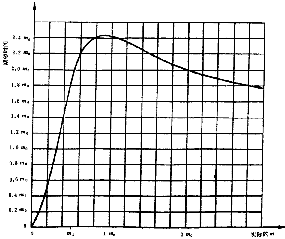
图 19 试验方案 4 : 6 判定的期望相关试验时间
