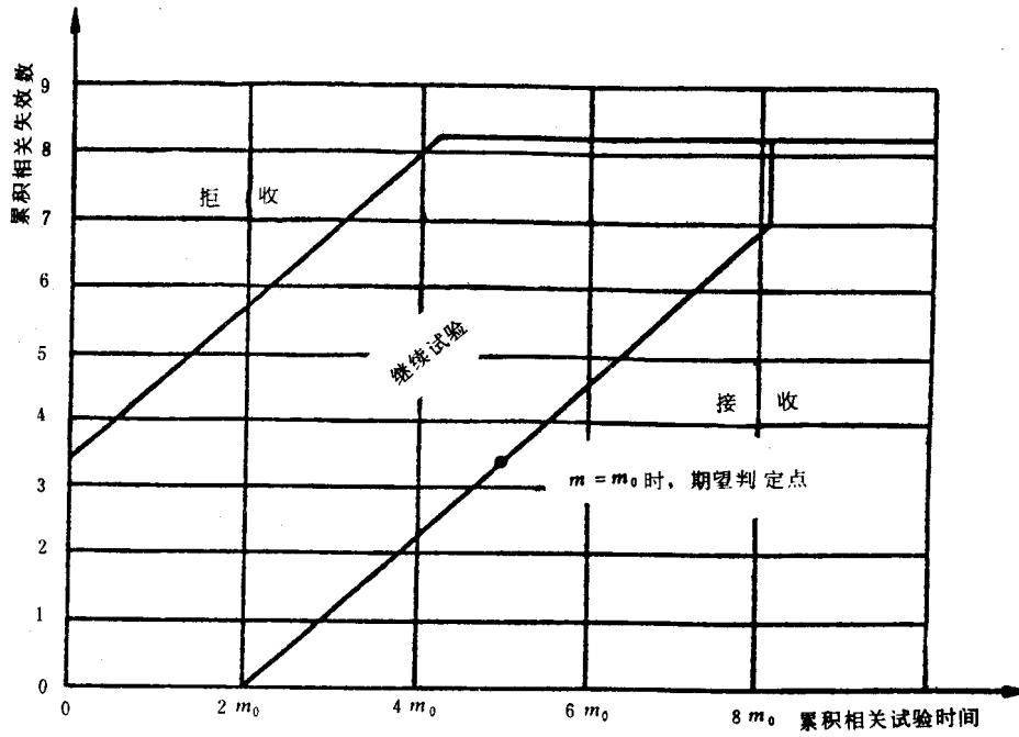
图 29 试验方案 4 : 10 ( \alpha=0.35, \beta=0.40, D_m=1.25 )
