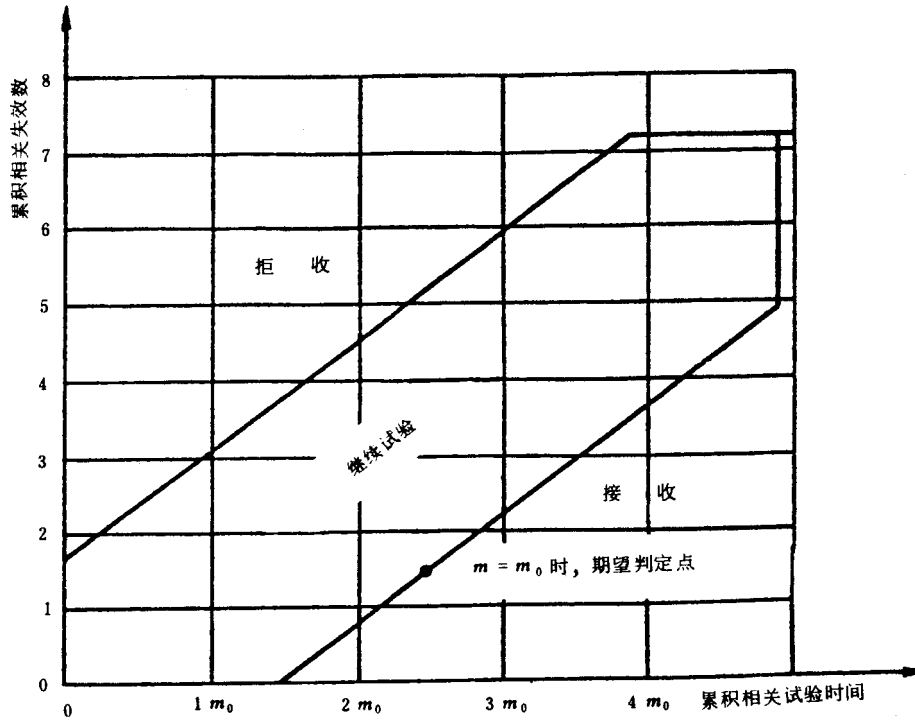
图 17 试验方案 4 : 6 ( \alpha=0.20, \beta=0.20, D_m=2.0 )
