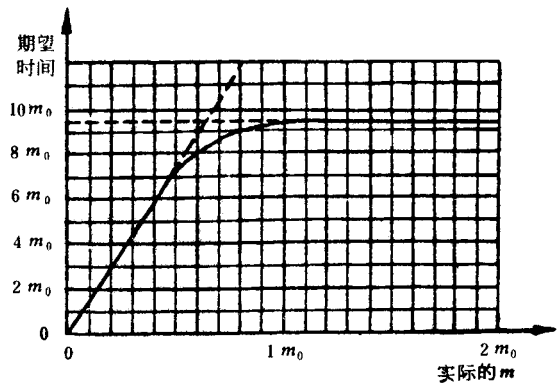
图 34 试验方案 5:2 判定的期望相关试验时间
