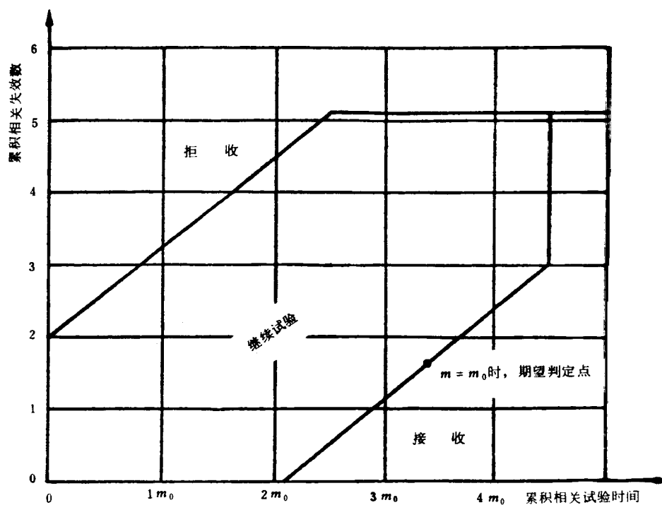
图 23 试验方案 4 : 8 ( \alpha=0.30, \beta=0.30, D_m=1.5 )
