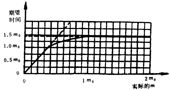
图 40 试验方案 5 : 7 判定的期望相关试验时间
