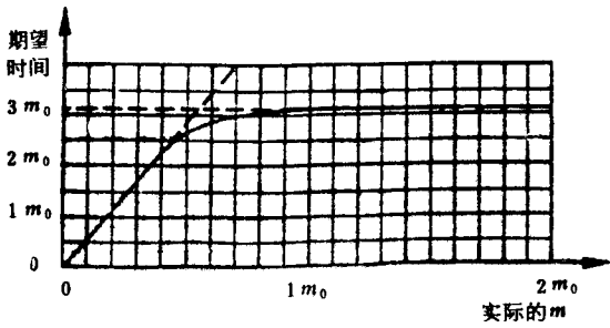
图 35 试验方案 5:3 判定的期望相关试验时间
