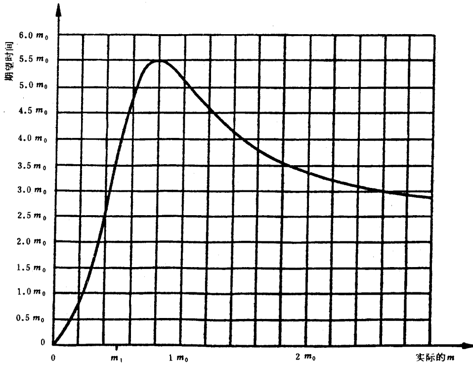
图 6 试验方案 4 : 2 工作特性曲线
