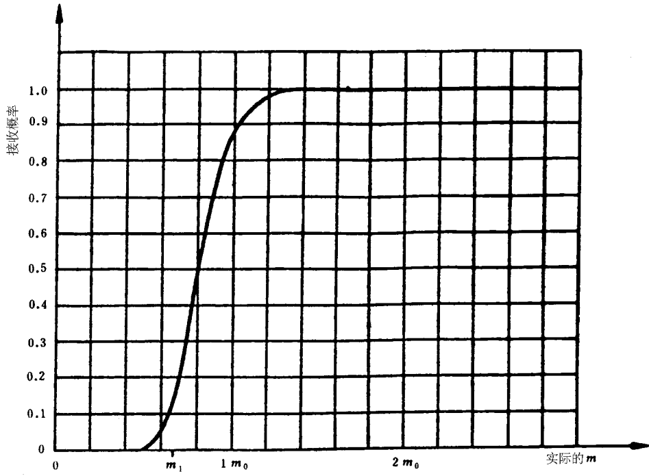
图 3 试验方案 4 : 1 工作特性曲线
