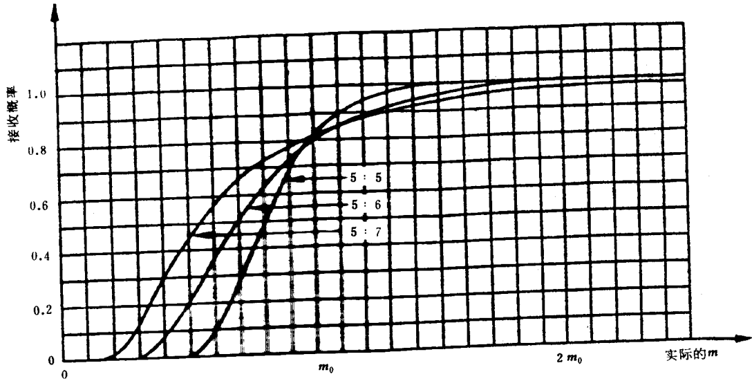
图 37 试验方案 5 : 5, 5 : 6, 5 : 7 工作特性曲线
