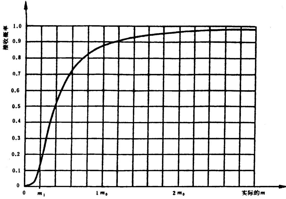
图 12 试验方案 4 : 4 工作特性曲线
