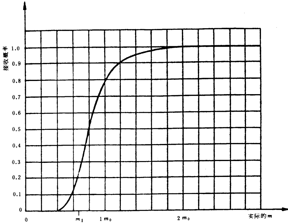
图 15 试验方案 4 : 5 工作特性曲线
